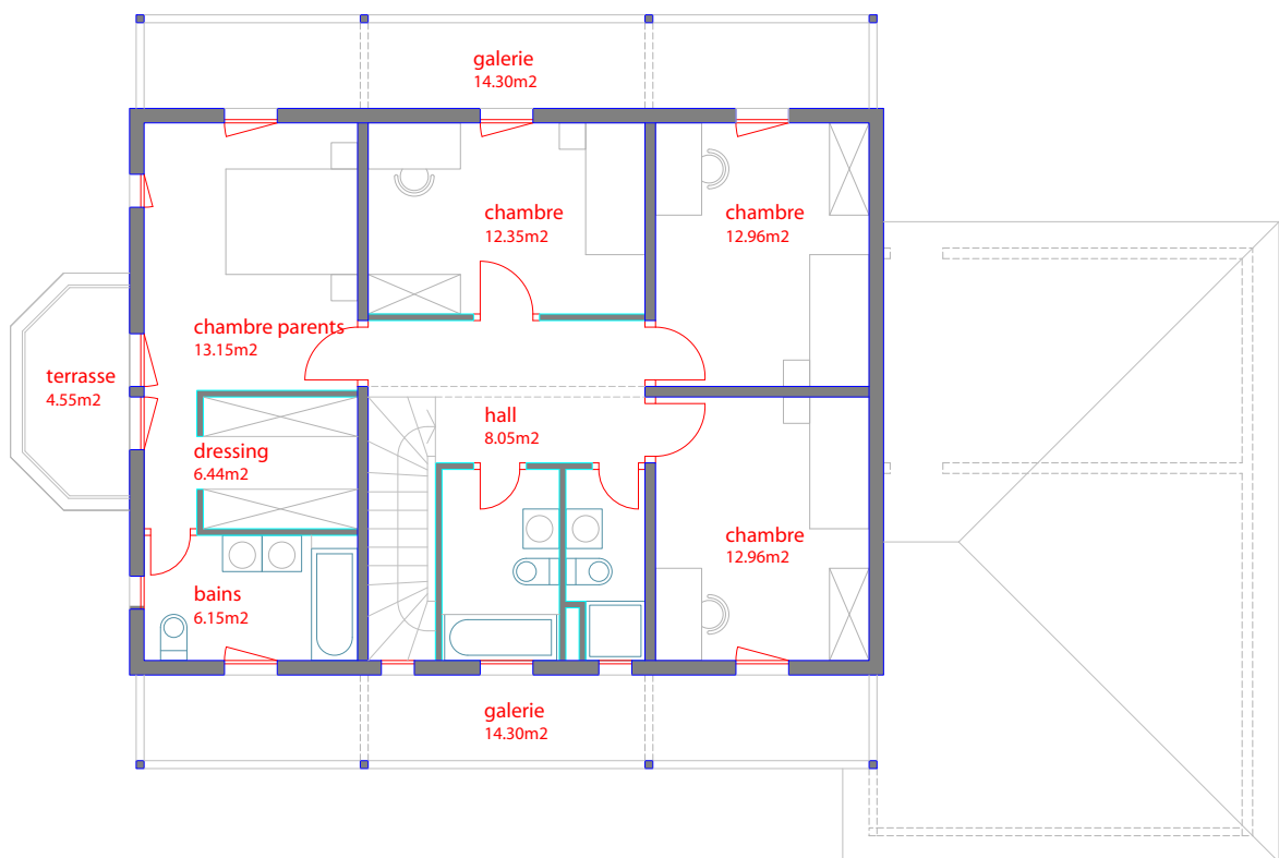
ETAGE 98 m 2
